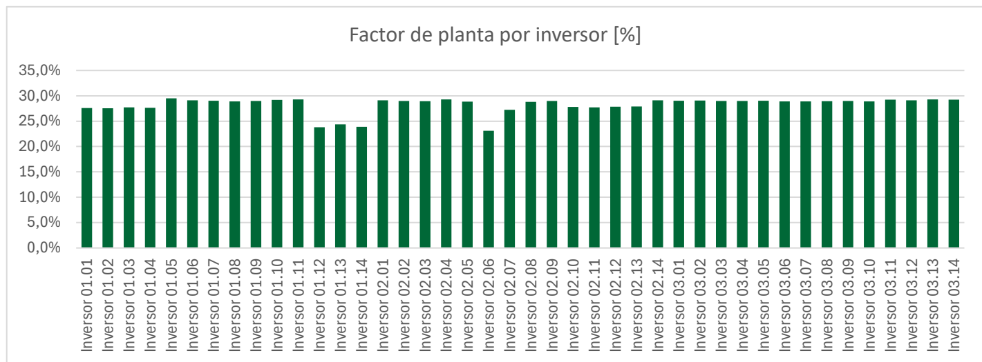
Gráfico N°2: Desempeño de Inversores.
