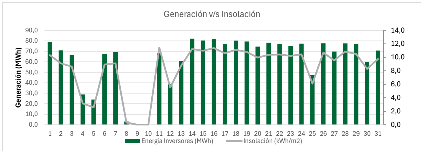
Grafico N°1: Generación v/s Insolación
